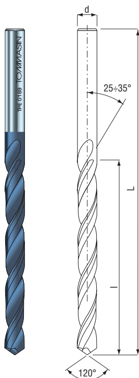
DIN 338
